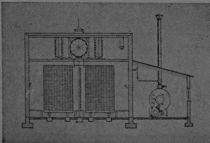
Equipo para el secado perfecto de madera con capacidad de 50.000 pulgadas.
